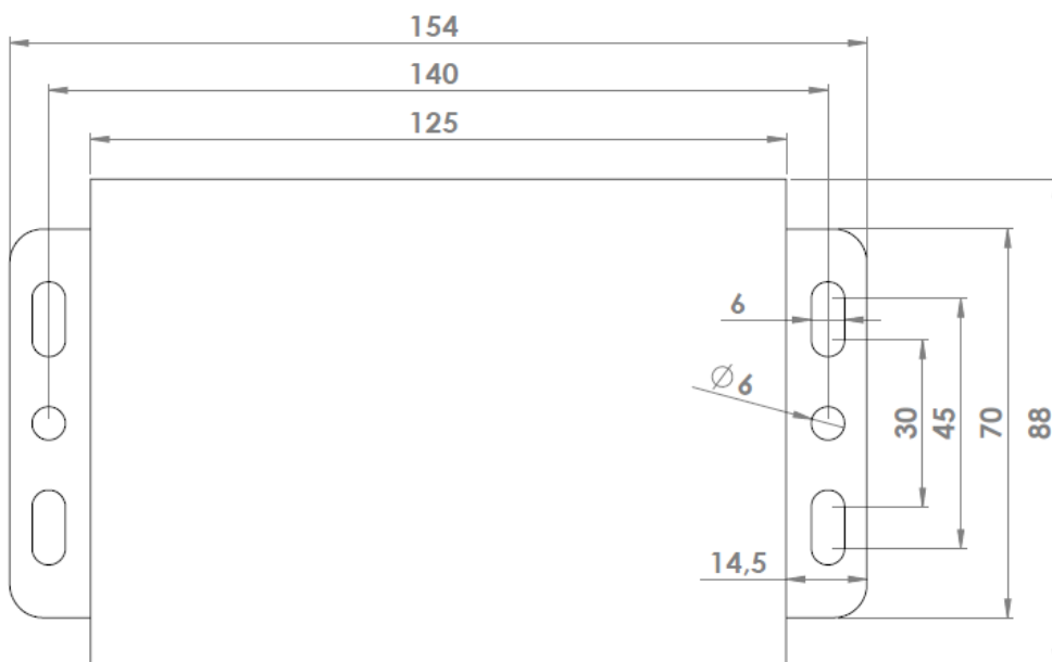
Abb.: Maße des Controllers
