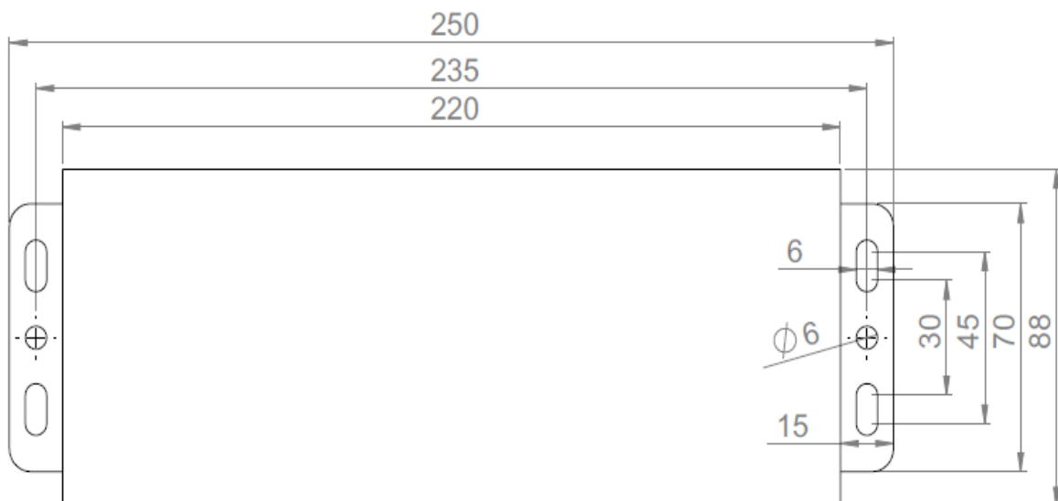
Abb.: Maße des Controllers
